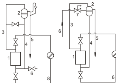
Rys. nr 8 Przykłady podłączenia otwartych zbiorników rozprężnych
