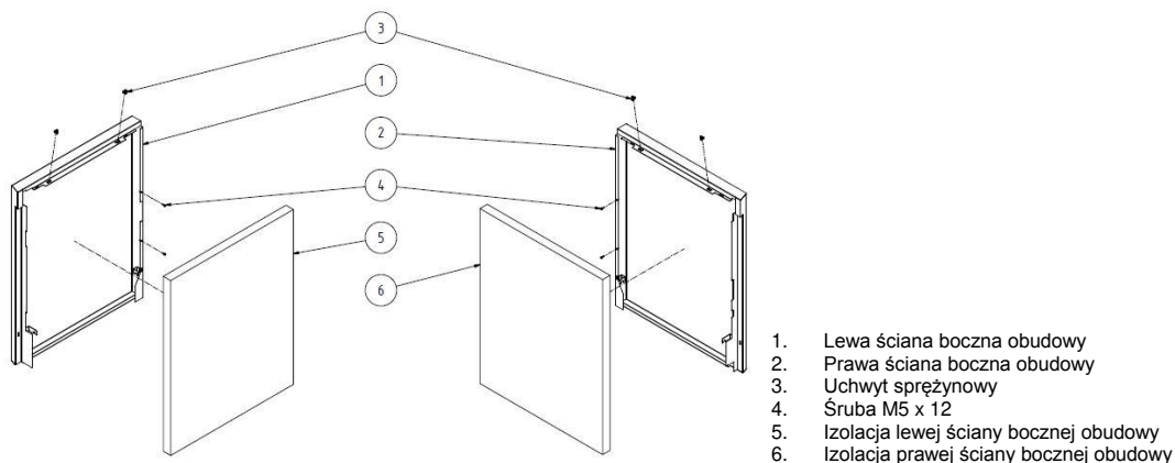
Rys. nr 20 Ściany boczne obudowy
