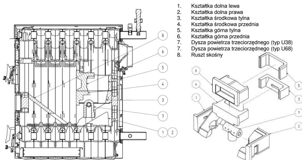
Rys. nr 16 Ulokowanie kształtek w komorze spalania kotła HERCULES U68, HERCULES U38
