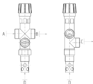
Rys. nr 6 Dwudrożny zawór bezpieczeństwa DBV 1 - 02
