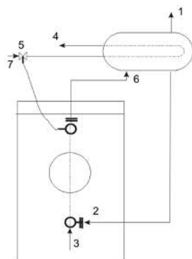
Rys. nr 5 Schemat hydrauliczny podłączenia pętli chłodzącej
