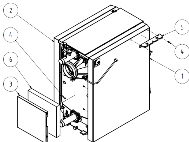
Rys. nr 23 Montaż części tylnej obudowy i uchwytu narzędzi do czyszczenia
