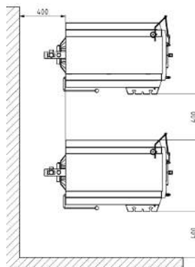
Rys. nr 12 Umiejscowienie kotłów w kotłowni
