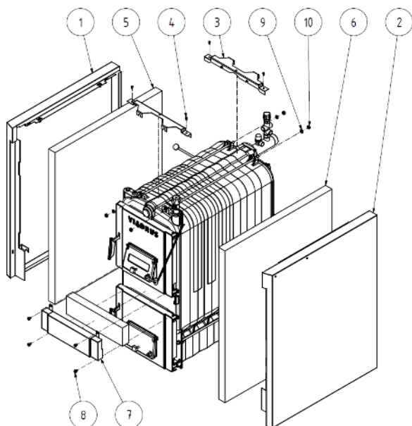
Rys. nr 21 Montaż ścian bocznych obudowy
