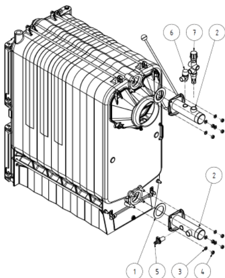
Rys. nr 13 Instalacja korpusu kotła
