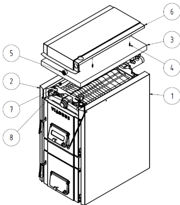
Rys. nr 22 Montaż części górnej obudowy
