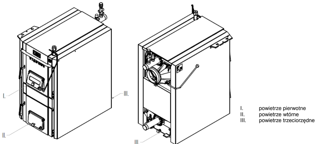
Rys. nr 27 Przepływ powietrza spalania
