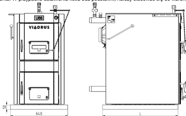
Rys. nr 10 Wymiary cokołu
