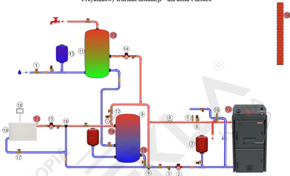
Przykładowy schemat instalacji – dla kotła Classico
